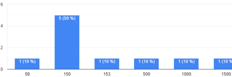
Réseaux Sociaux
